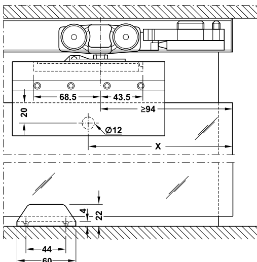
Trolley hanger and guide Bánh xe và dẫn hướng
