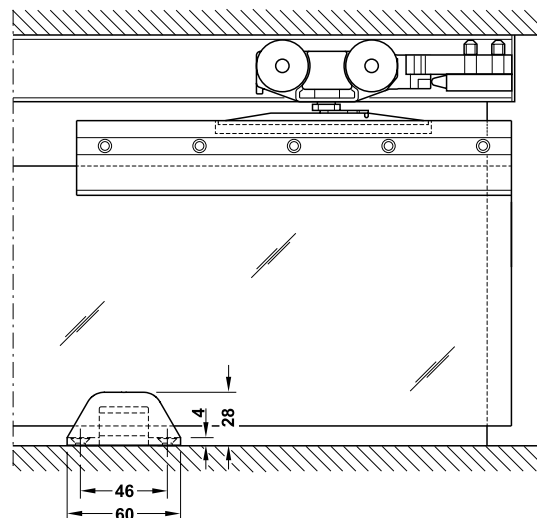
Guide and trolley hanger Dẫn hướng và bánh xe treo
